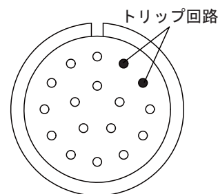
図11 ケーブル側コネクタから見た開閉器トリップ回路位置
