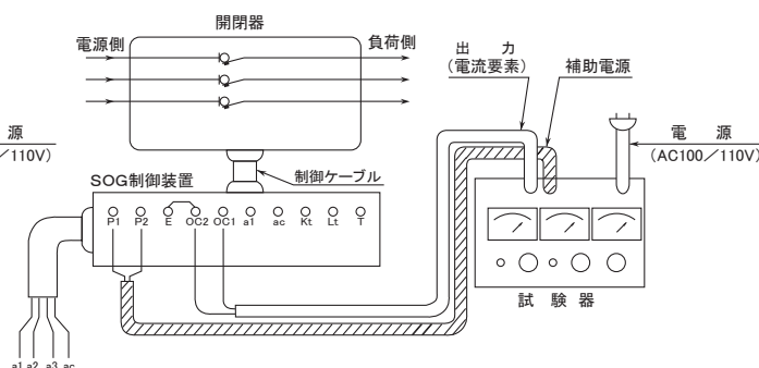
図7 ムサシインタック製(RDF) によるOCR動作特性チェック回路 ※クリップ色については試験器メーカーの取扱説明書などを ご参照ください。
