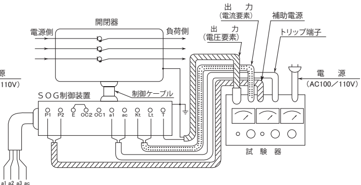
図5 ムサシインタック製(RDF)による地絡特性チェック回路
