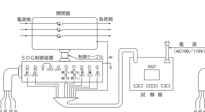
図4 戸上電機製作所製(DGT)による地絡特性チェック回路
