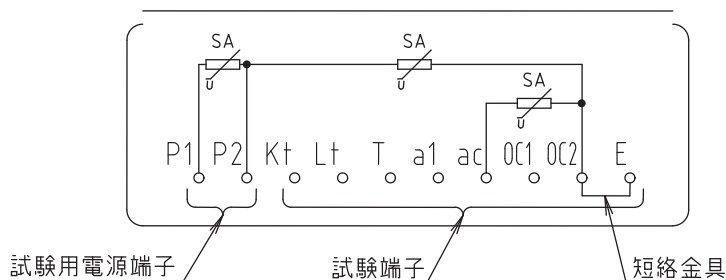
図2 SA(避雷器)の設置
