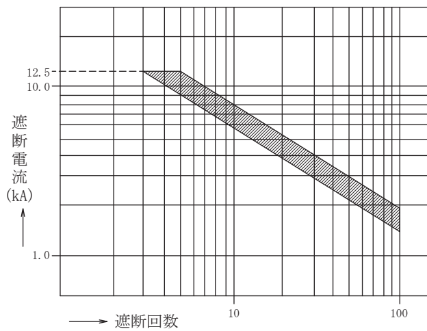
遮断電流－遮断回数特性
