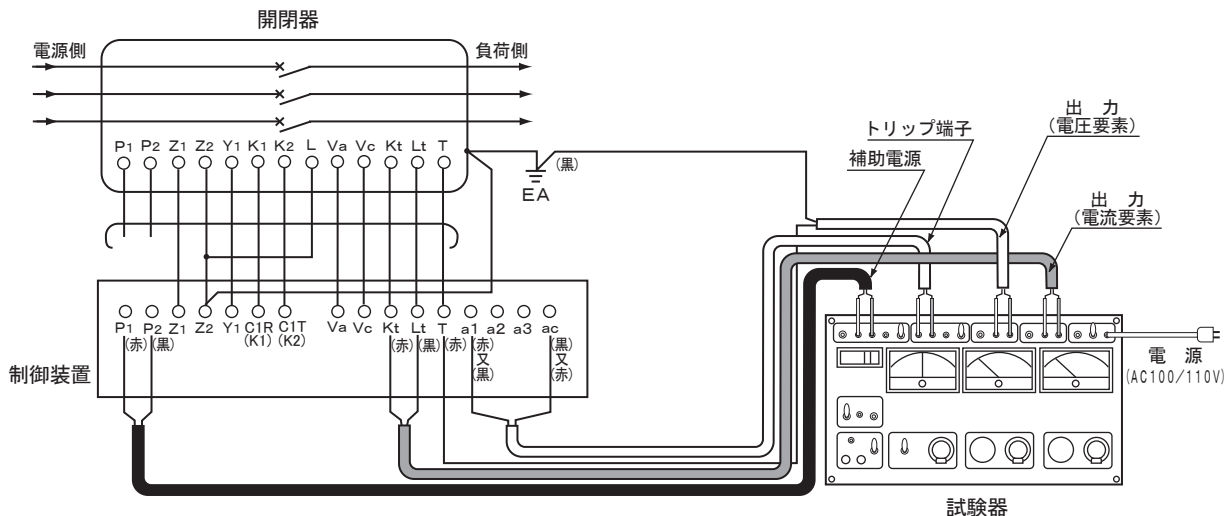
図10 双興電機製作所製(DGR)によるテスト回路の一例
