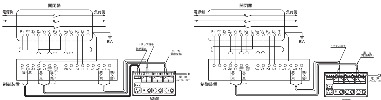
【図15-1 制御装置に電源が供給されていない場合】
