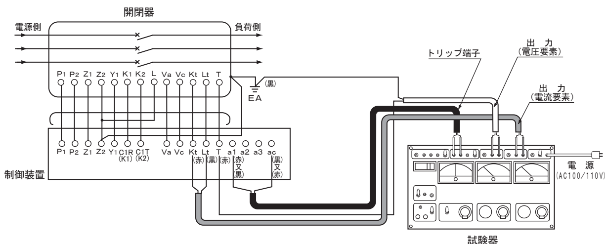
図11 双興電機製作所製(DGR)によるテスト回路の一例
