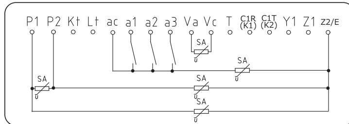
図9 SA(避雷器)の設置
