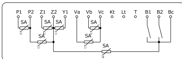
図20 サージアブソーバ(避雷器)の設置(1回路用屋外形・表面形)
