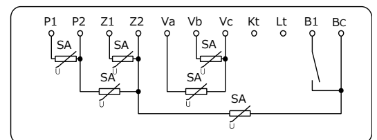
図21 サージアブソーバ(避雷器)の設置
