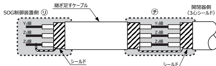
図11 ケーブルの継ぎ足し (当社で取扱いの3心一括シールド付ケーブルをご使用の時)
