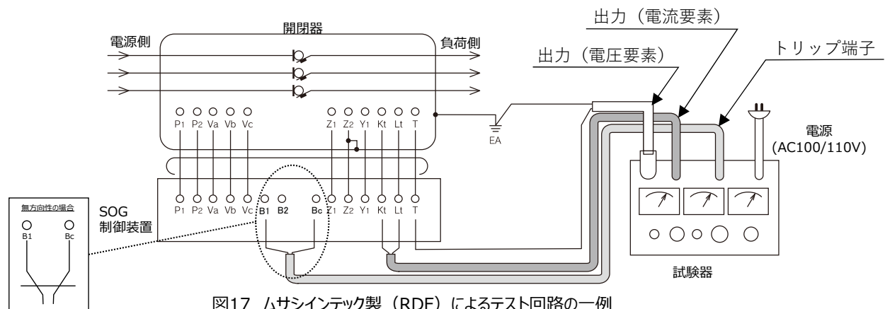
図17 ムサシインテック製（RDF）によるテスト回路の一例
