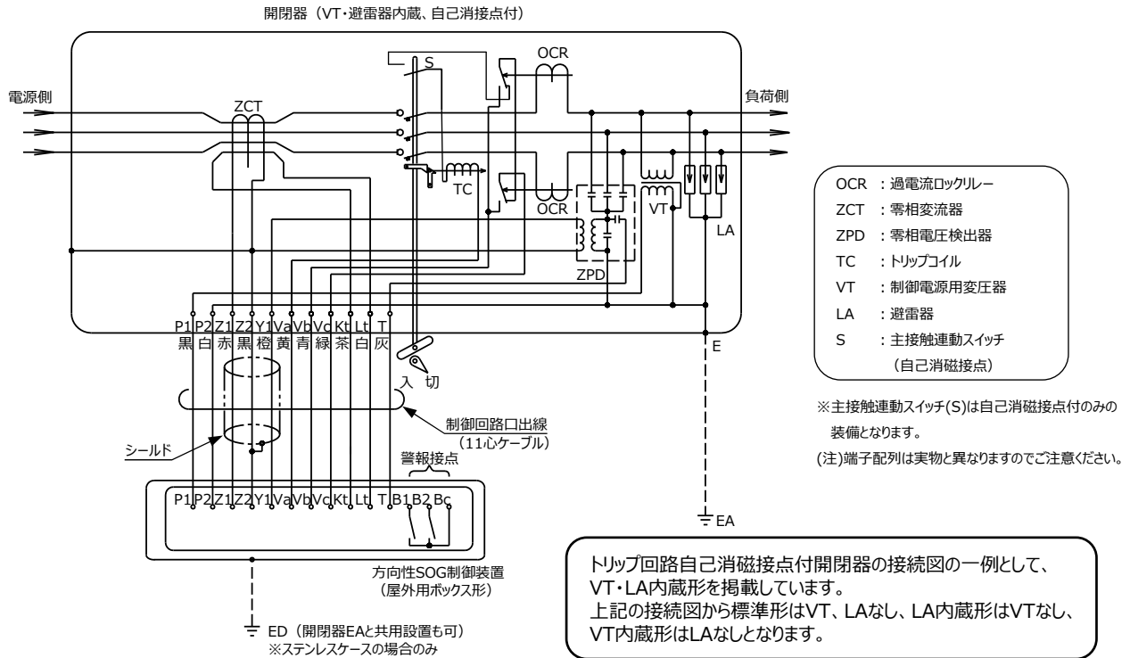
トリップ回路自己消磁接点付 方向性 VT・LA内蔵形 接続図
