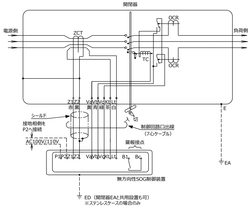
無方向性 LA内蔵形 接続図
