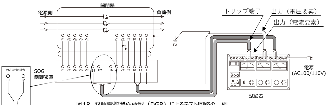
図18 双興電機製作所製（DGR）によるテスト回路の一例
