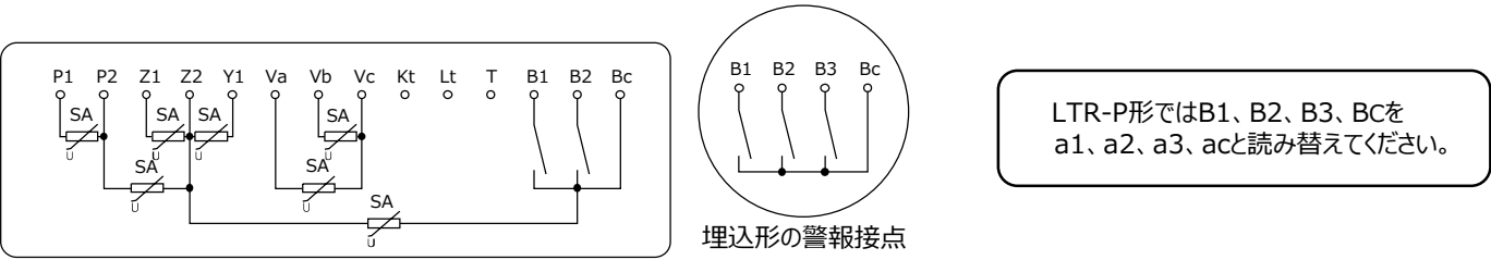
図 1 9 サージアブソーバ（避雷器）の設置（1回路用屋外形・表面形）
