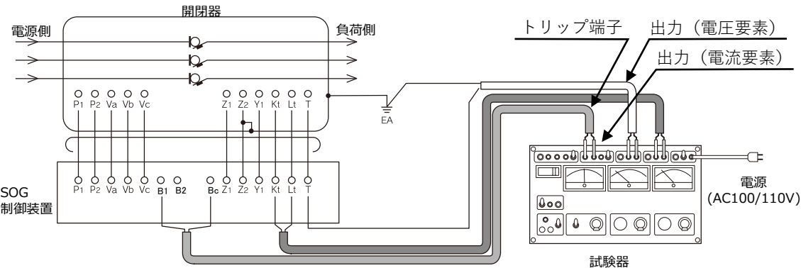
図 1 7 双興電機製作所製（DGR）によるテスト回路の一例
