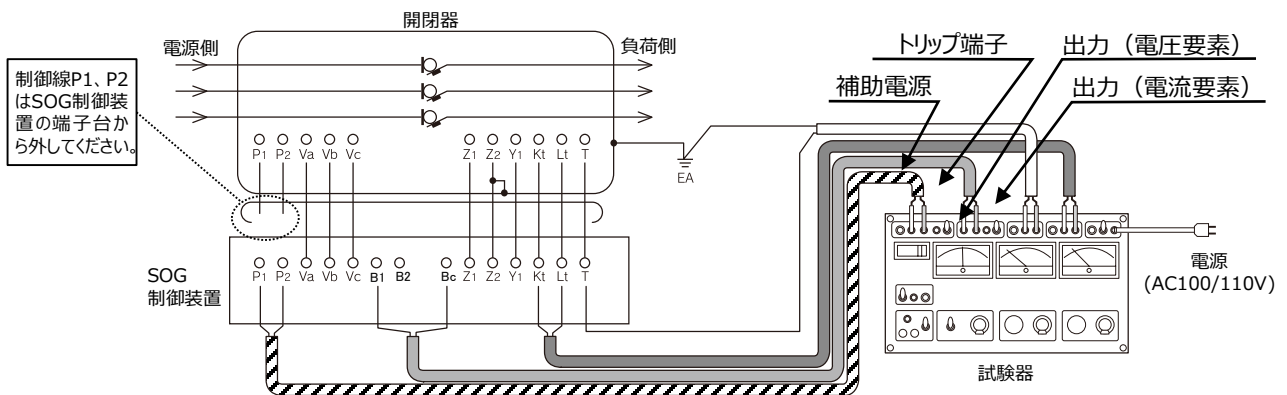
図1 4 双興電機製作所製（DGR）によるテスト回路の一例
