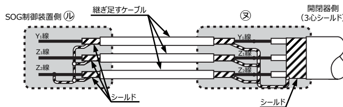
図11 ケーブルの継ぎ足し (お客様で単独シールド付電線をご使用の時)
