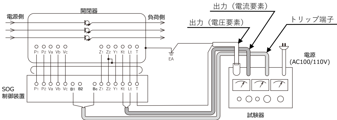
図 1 6 ムサシントック製（RDF）によるテスト回路の一例
