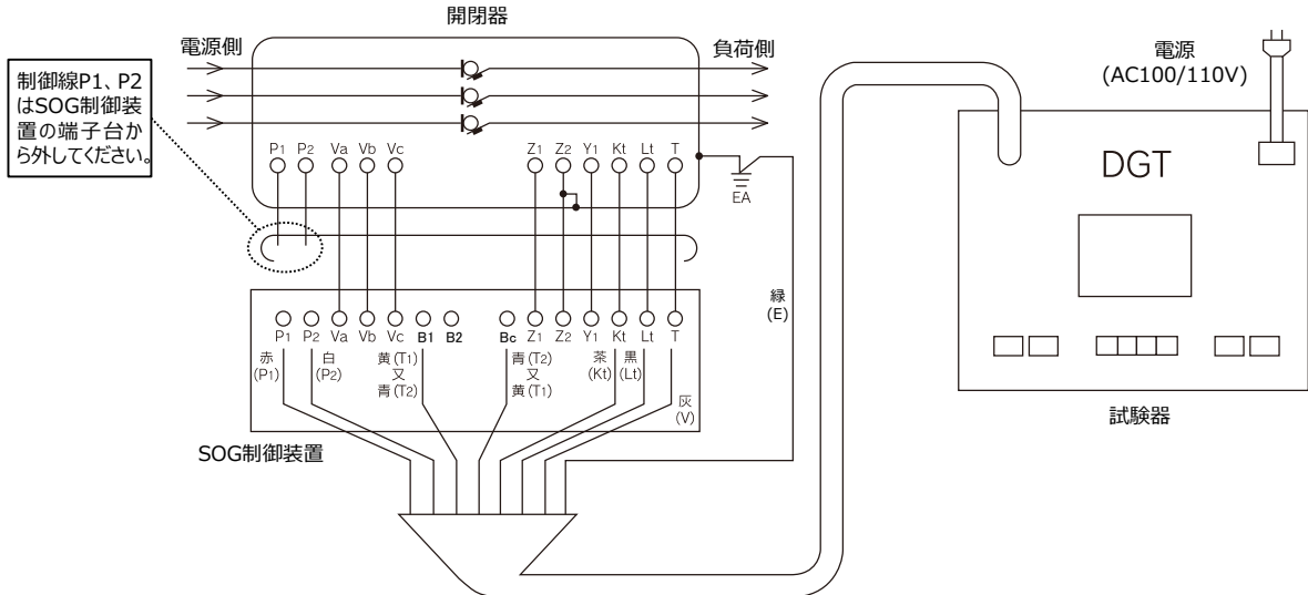
図1 2 戸上電機製作所（DGT）によるテスト回路の一例
