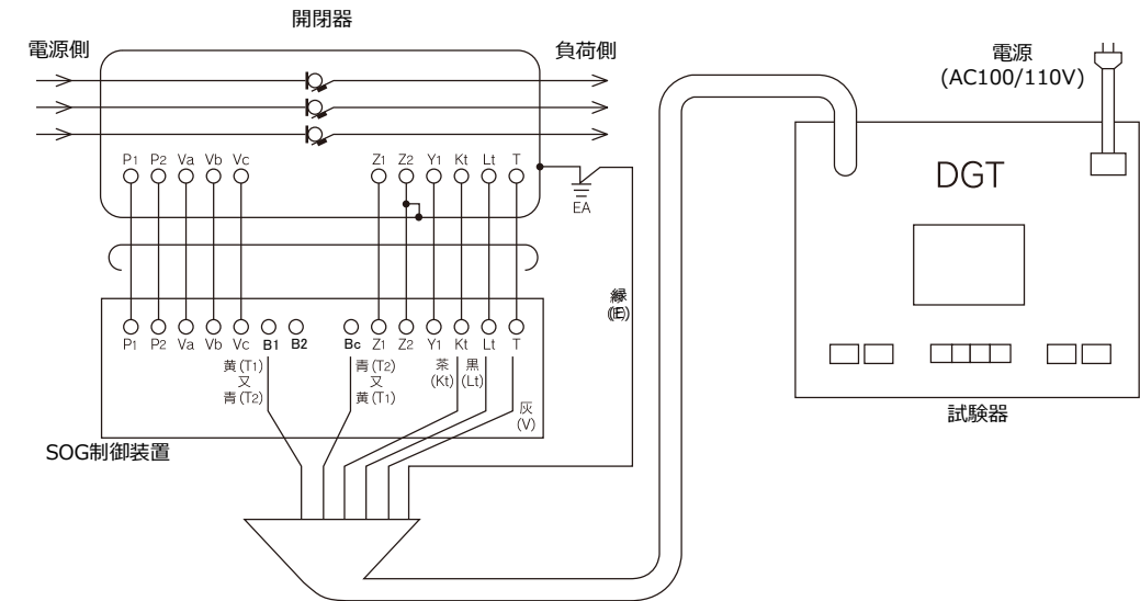
図 1 5 戸上電機製作所（DGT）によるテスト回路の一例
