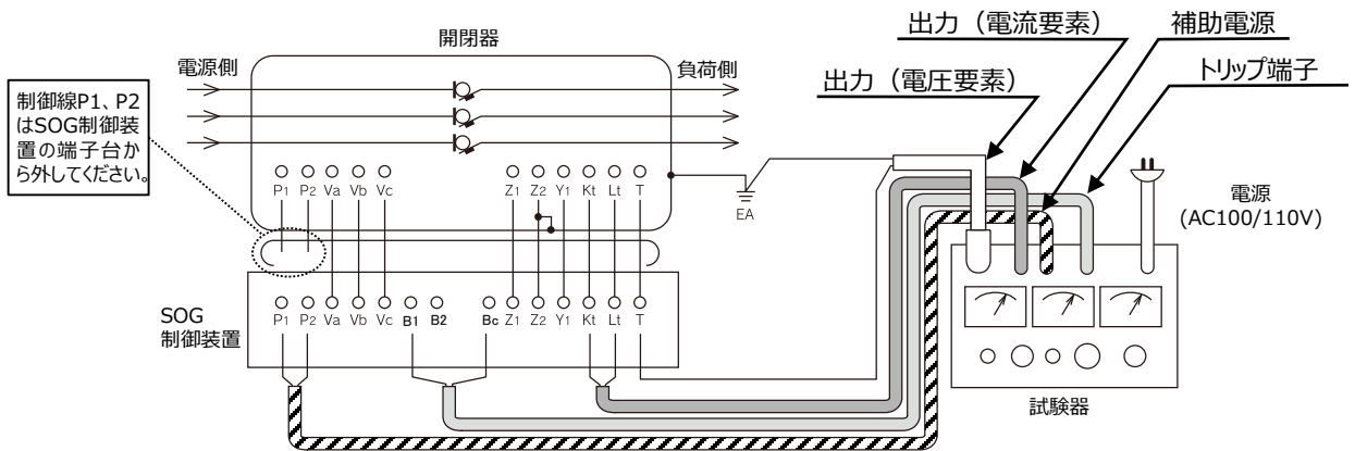
図1 3 ムサシントック製（RDF）によるテスト回路の一例
