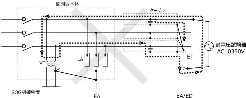
図1 8 一相のみに試験電圧を印加した場合の電流経路
