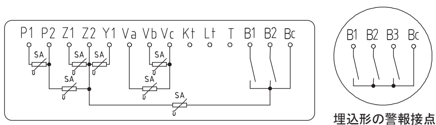
図11 SA(避雷器)の設置
