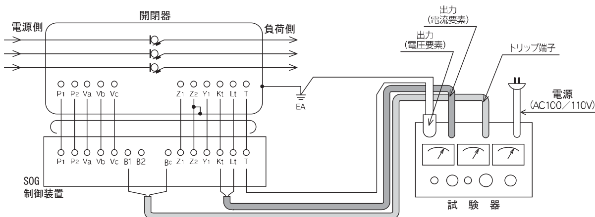
図 16 ムサシインテック製(RDF)によるテスト回路の一例
