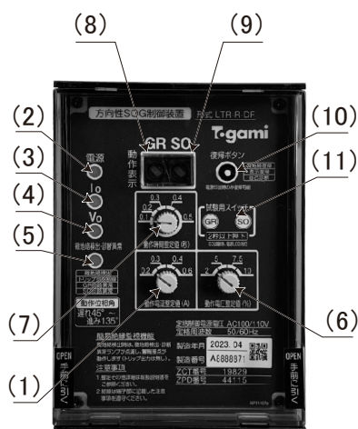
埋込形(LTR-R-DF)
