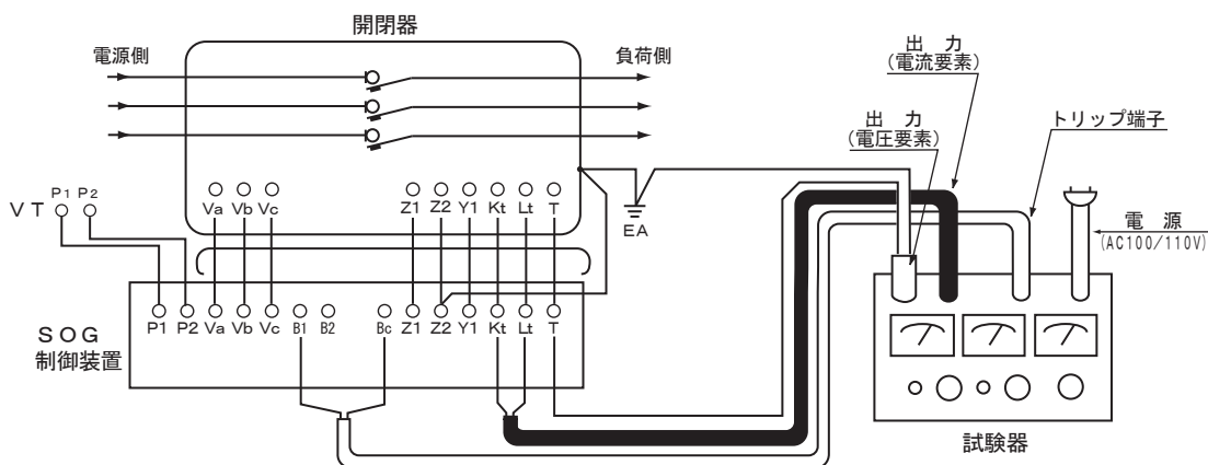
ムサシインテック製(RDF)によるテスト回路の一例
