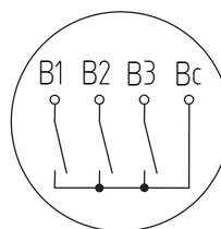
埋込形の警報接点
