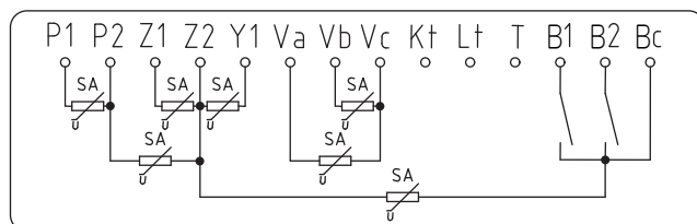
SA(避雷器)の設置 [表面形]
