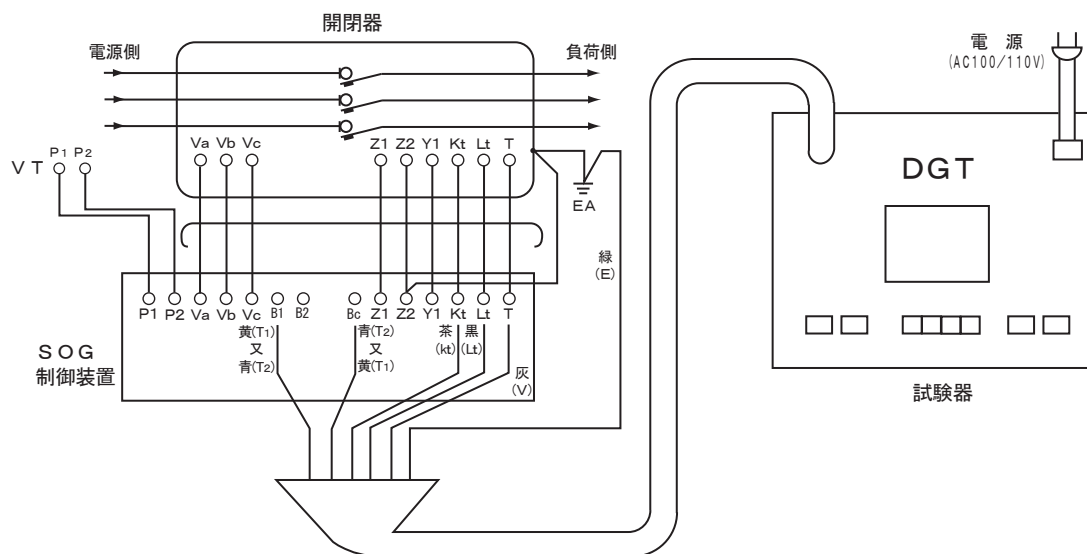
戸上電機製作所製(DGT)によるテスト回路の一例
