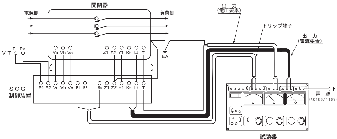
双興電機製作所製(DGR)によるテスト回路の一例
