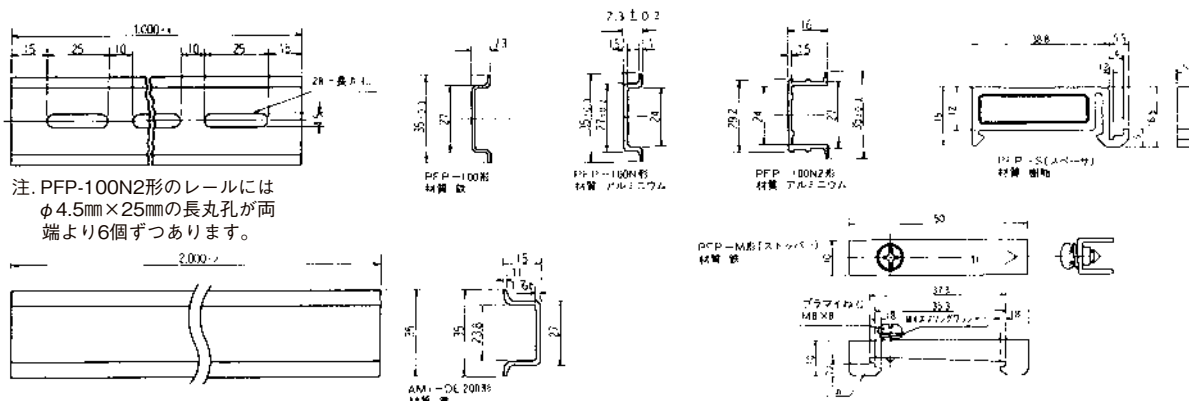
正規取付
