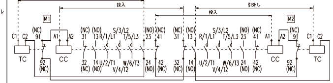
接点構成
