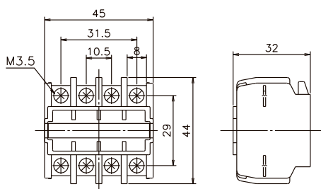
HAU-4 (4P形)
