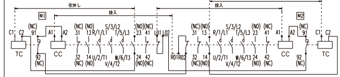
接点構成
