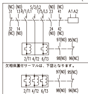
PAK-26JT~50JT-SL2(C) PAK-26JGT~50JGT-SL2(C)
