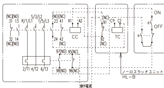
PAK-50HTC~95HTC
