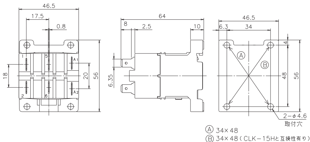
電磁接触器 CLK-25JF2
