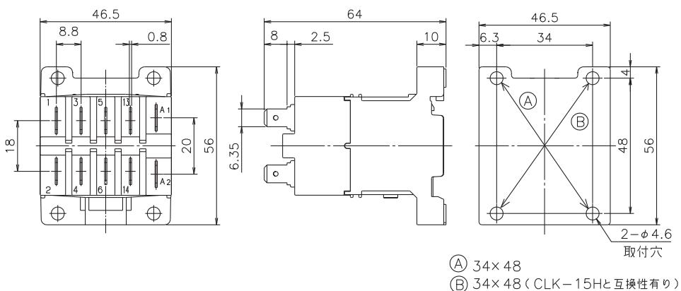
電磁接触器 CLK-15JFC
