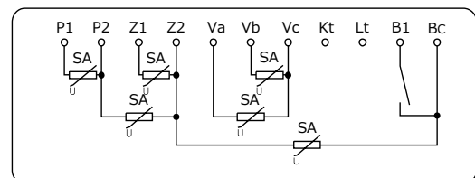
図21 サージアブソーバ(避雷器)の設置
