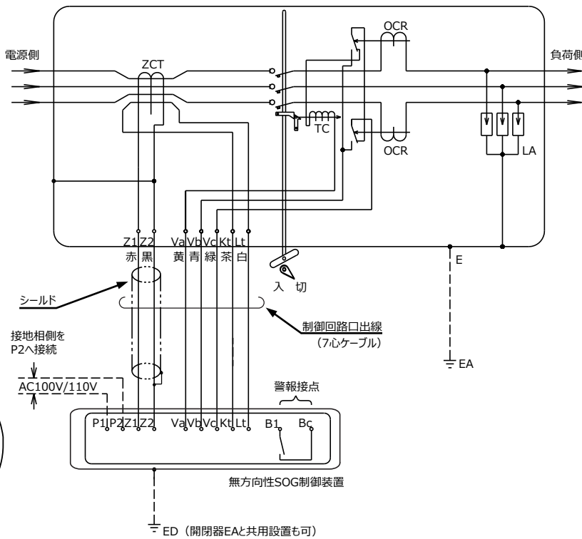
開閉器 (避雷器内蔵)
