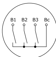
埋込形の警報接点
