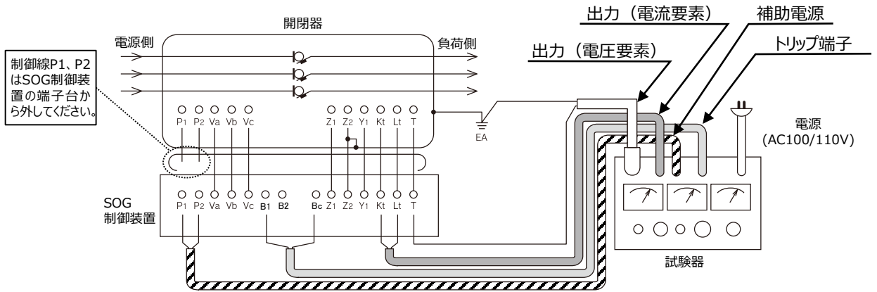
図1 3 ムサシントック製 (RDF) によるテスト回路の一例 ※クリップ色については試験器メーカーの取扱説明書などをご参照ください。
