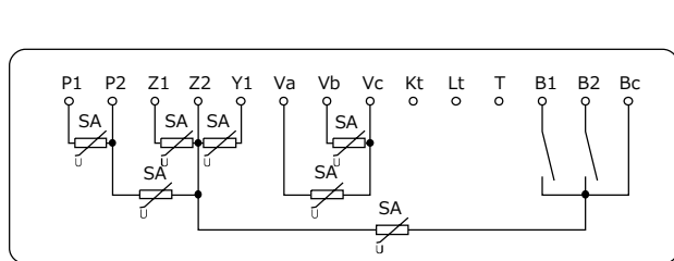
図19 サージアブソーバ(避雷器)の設置(1回路用屋外形・表面形)
