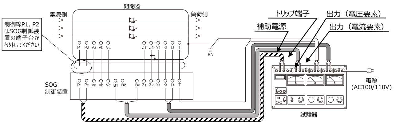
図1 4 双興電機製作所製 (DGR) によるテスト回路の一例 ※クリップ色については試験器メーカーの取扱説明書などをご参照ください。
