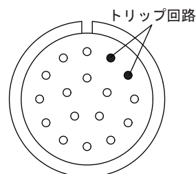
図5 ケーブル側コネクタから見た開閉器トリップ回路位置
