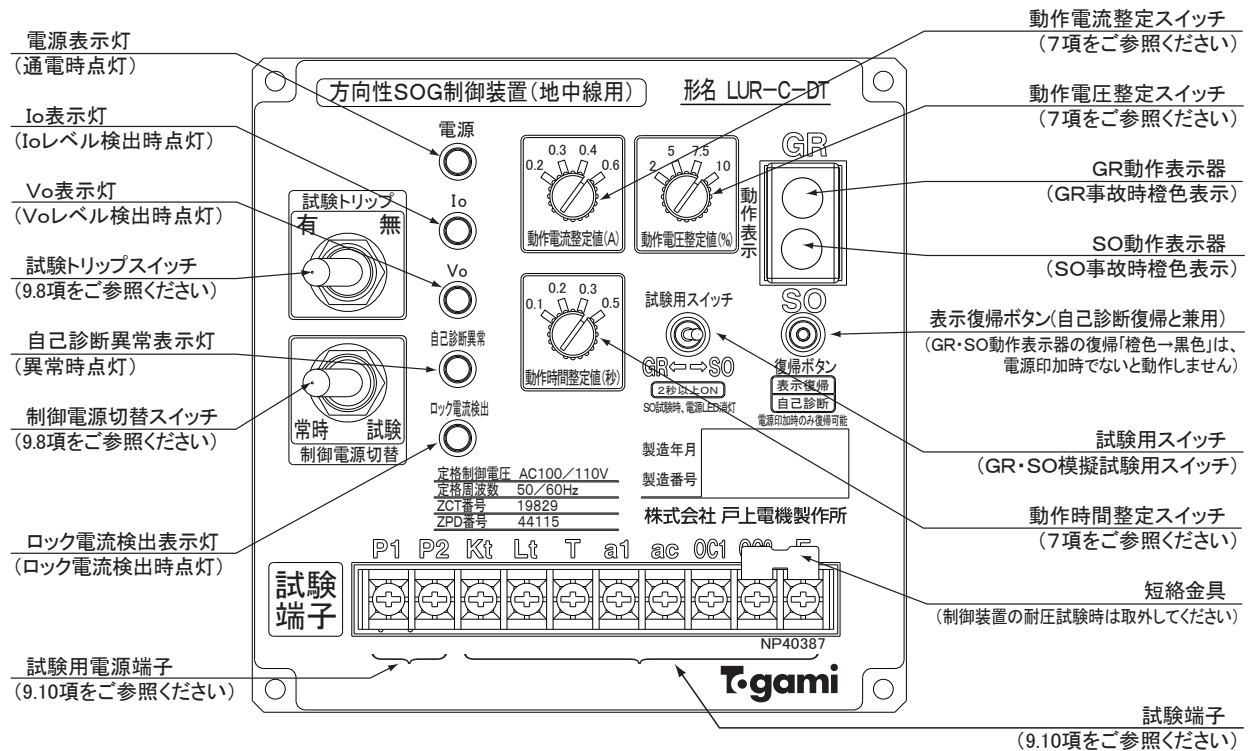
図 2 制御装置パネル面
