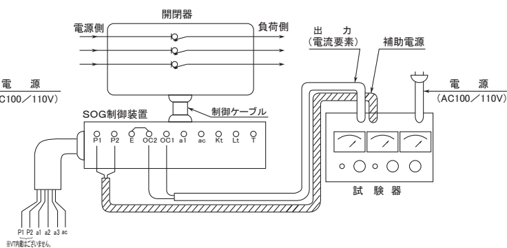
図8 ムサシインタック製(RDF)による OCR動作特性チェック回路
