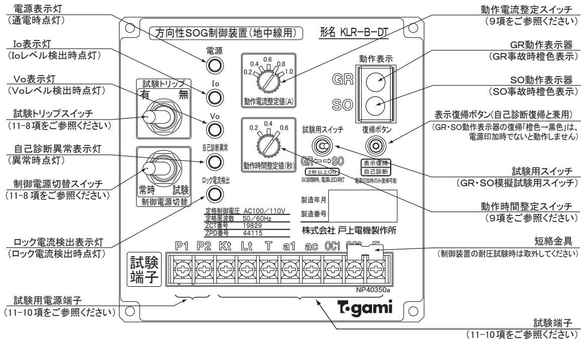
図 4 制御装置パネル面
