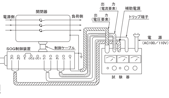
図6 ムサシインタック製(RDF)による 地絡特性チェック回路
