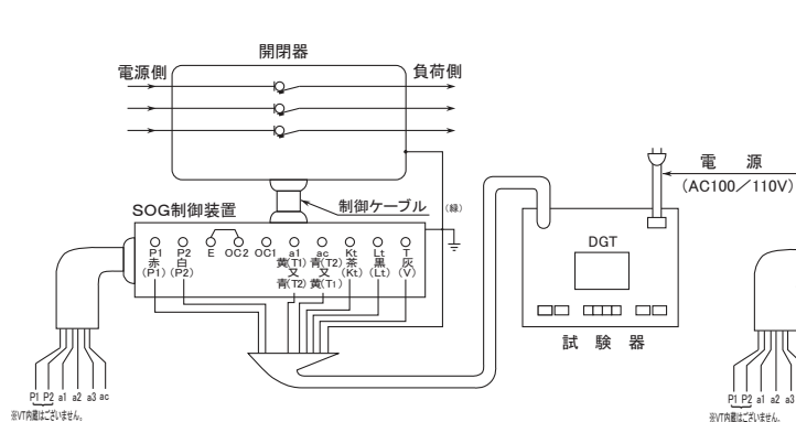
図5 戸上電機製作所製(DGT)による 地絡特性チェック回路
