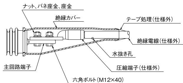
主回路端子部構造(上面図)
