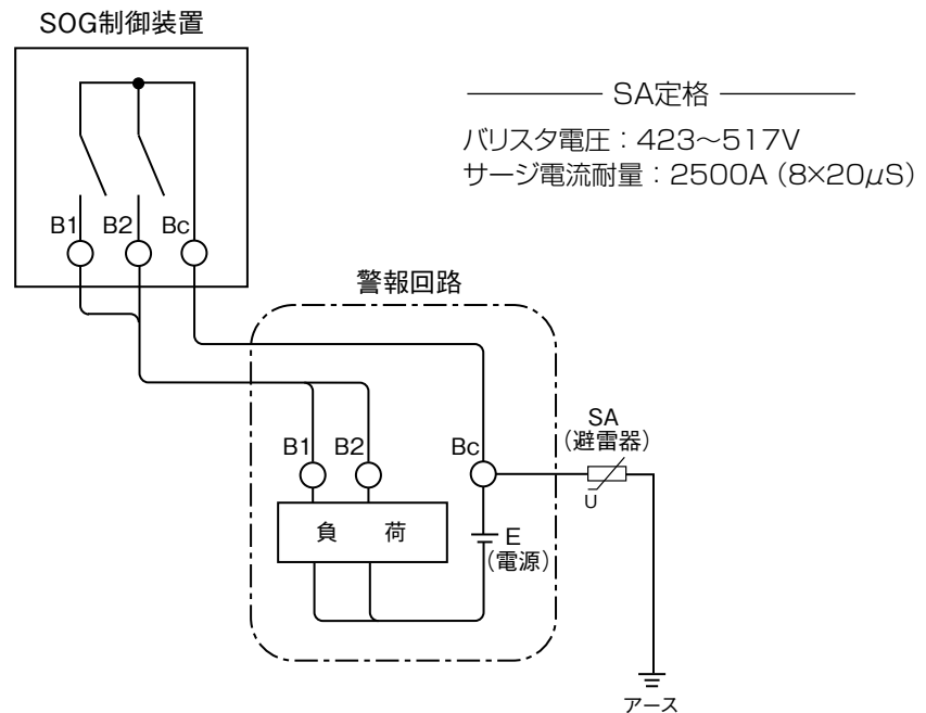
[方向性の場合の回路例]
